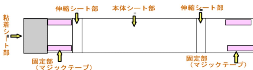
材料構成（イメージ図）
