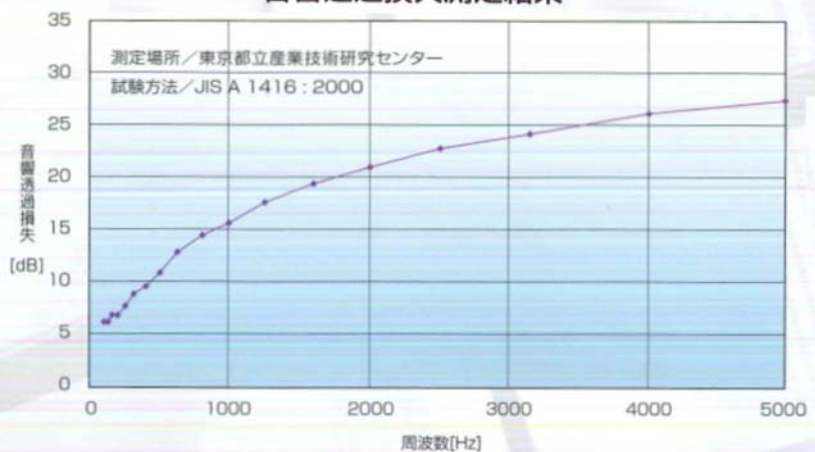
音響透過損失測定結果
