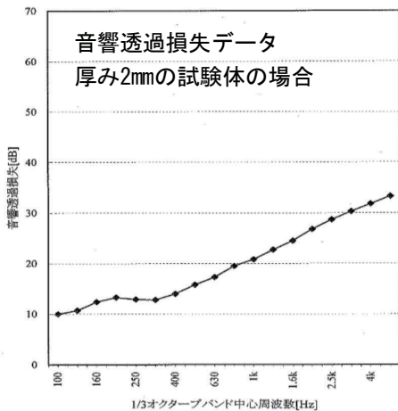
防音オールクリア 3Sの音響透過損失のテスト (2013年8月23日 東京の公的試験機関で実施)
