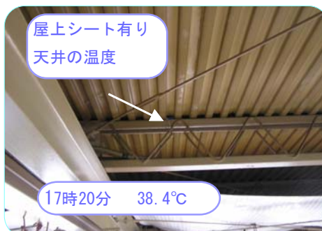
施工例：工場屋根 遮熱シート
