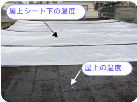
施工例：工場屋根 遮熱シート
